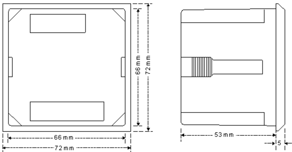
背視圖
